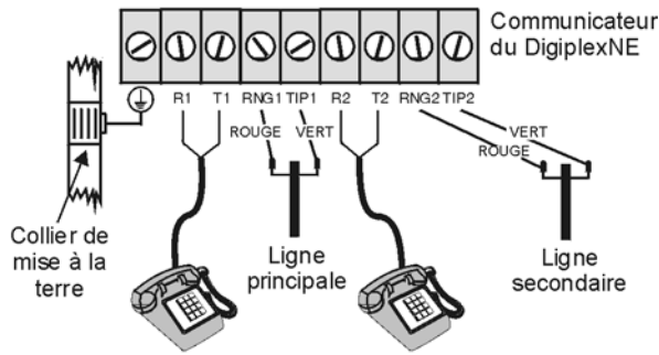
Figure 2-10 : Exemples de raccordement des lignes téléphoniques Exemple 1 :
