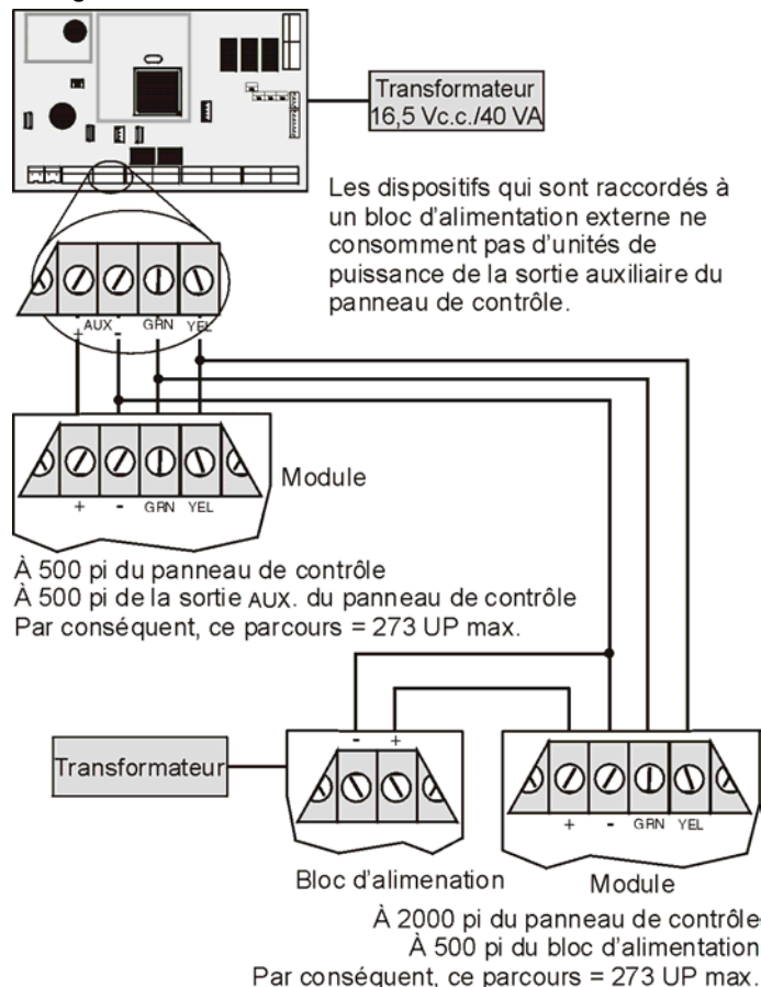
Figure 2-5 : Raccordement d'un bloc d'alimentation externe
