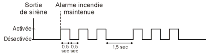
Figure 4-4 : Sortie de cloche/sirène durant une alarme incendie
