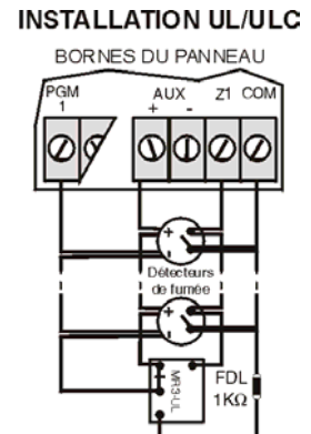
Figure 2-9 : Détecteurs à 4 fils
