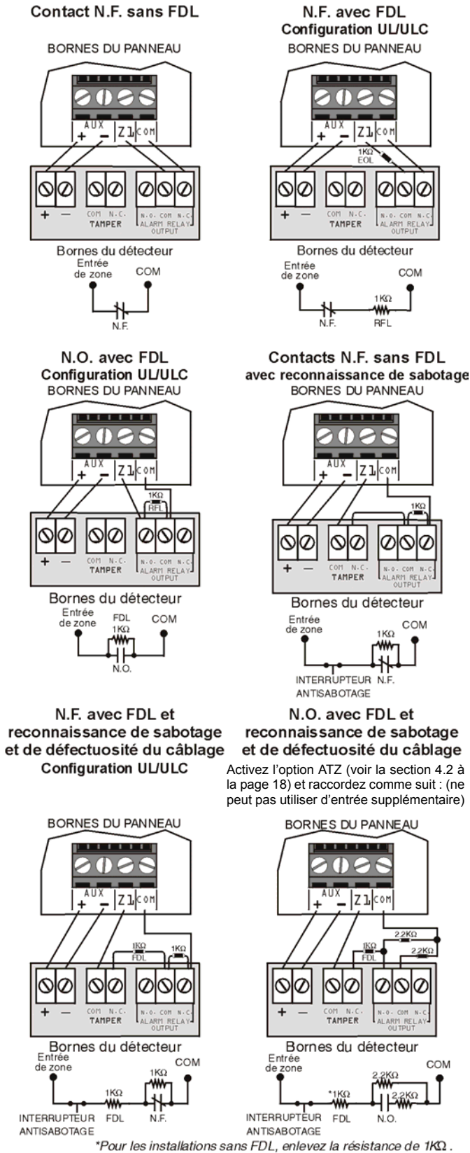
Figure 2-6 : Raccordement d'une zone simple
