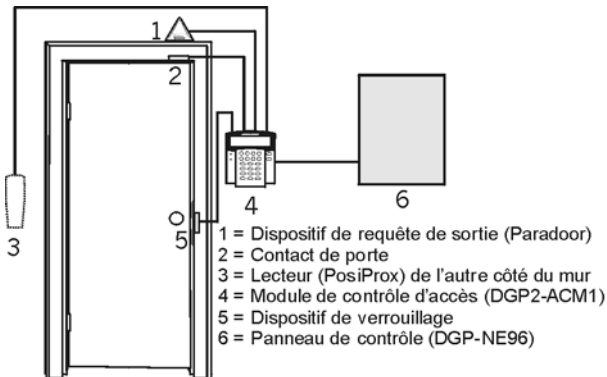
Figure 13-1 : Installation de contrôle d'accès typique*
