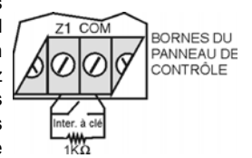
Figure 2-2 : Interrupteur
